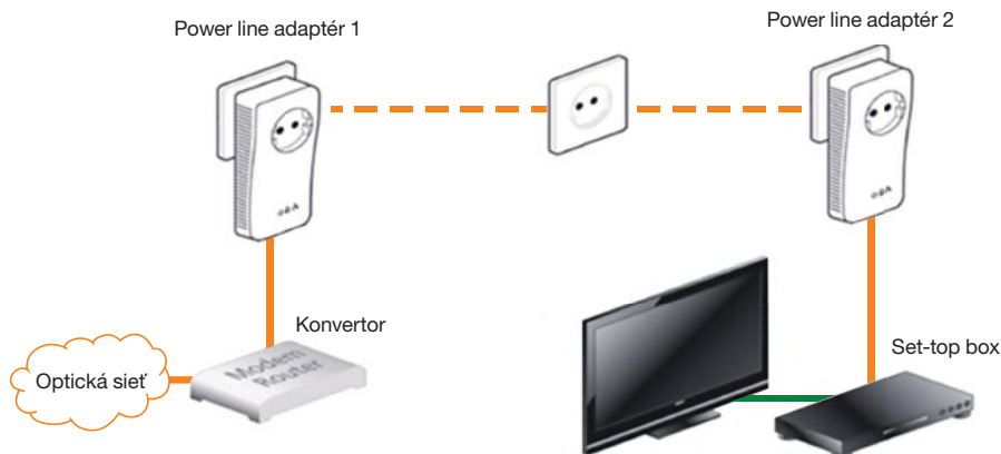
Obrázok č. 3 – pripojenie cez Power line adaptéry
